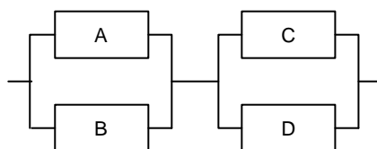
圖 5：四元件並串混聯系統可靠度方塊圖
