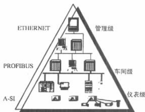
图 2 流程工业的一般网络体系
